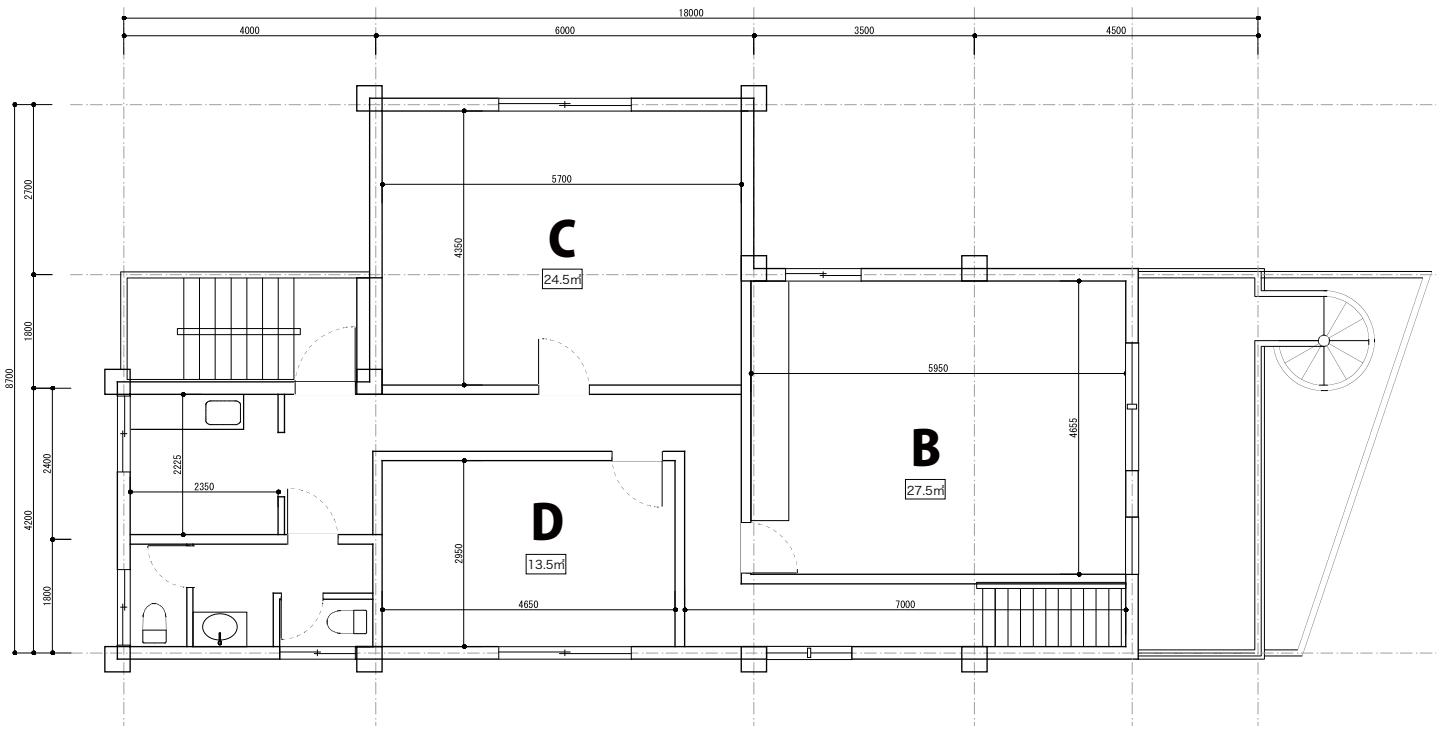
3階平面図
