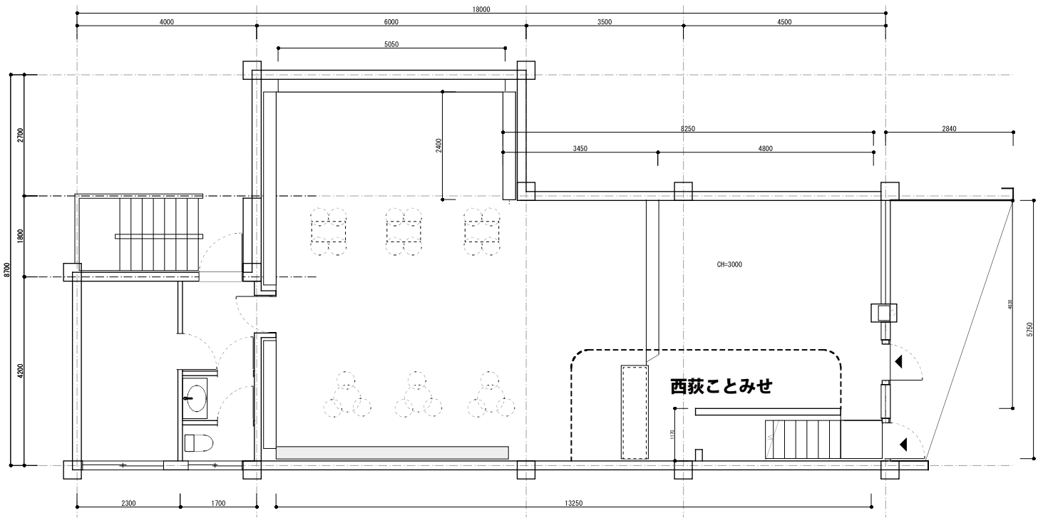
1階平面図
